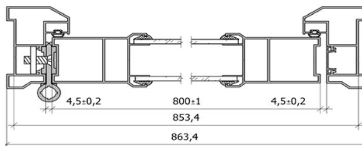
Схема 1. Крепление двери
