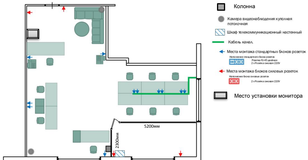
Схема 2. Помещение для монтажа/демонтажа оборудования
